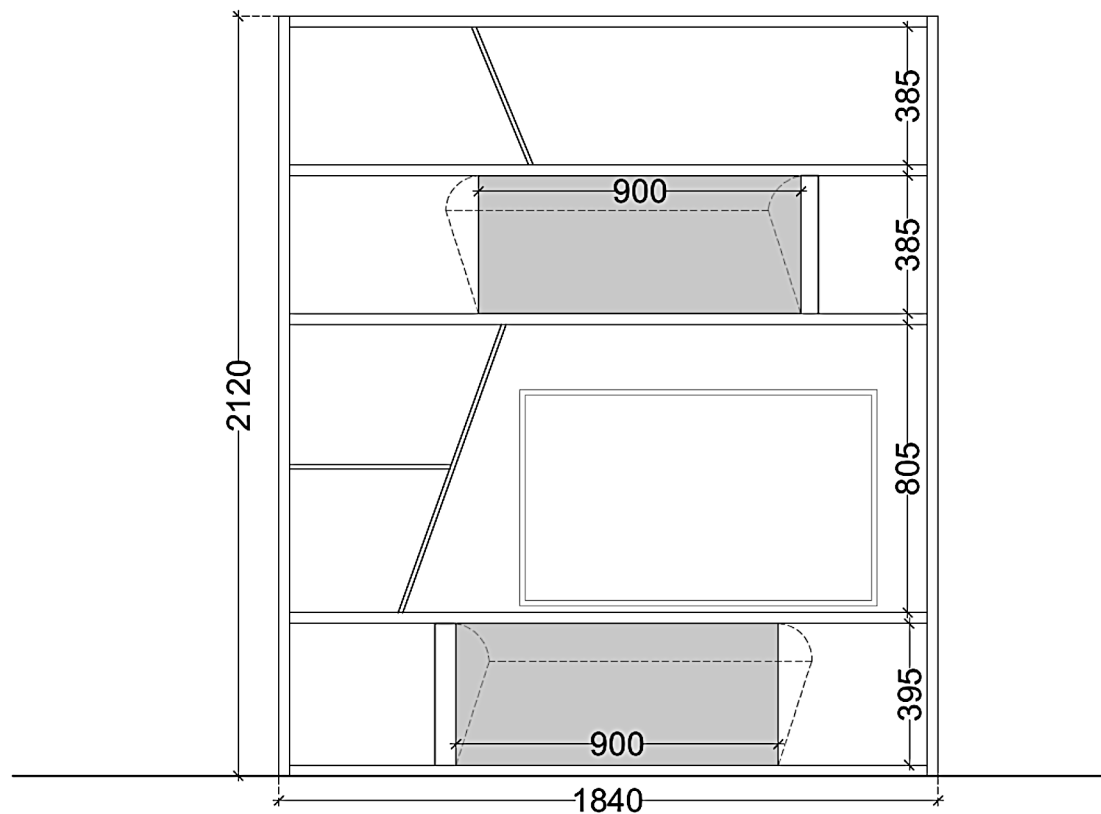
PROSPETTO
