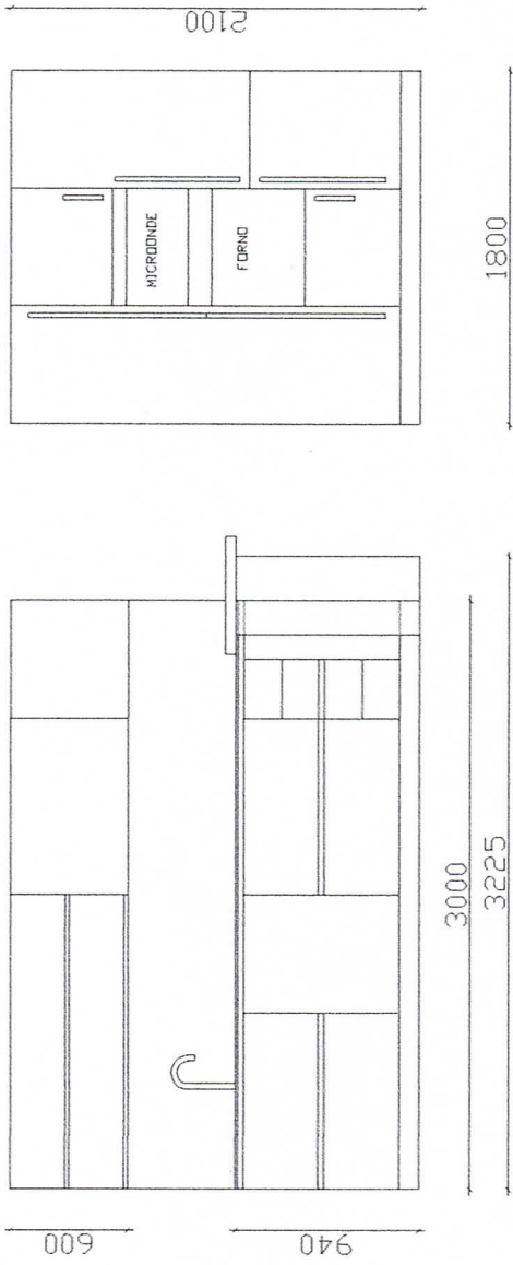
SEZIONE FRONTALE CUCINA
